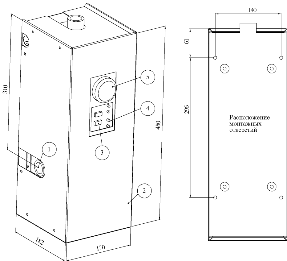
Рис. 1 Внешний вид электрокотла «MiniStar».
