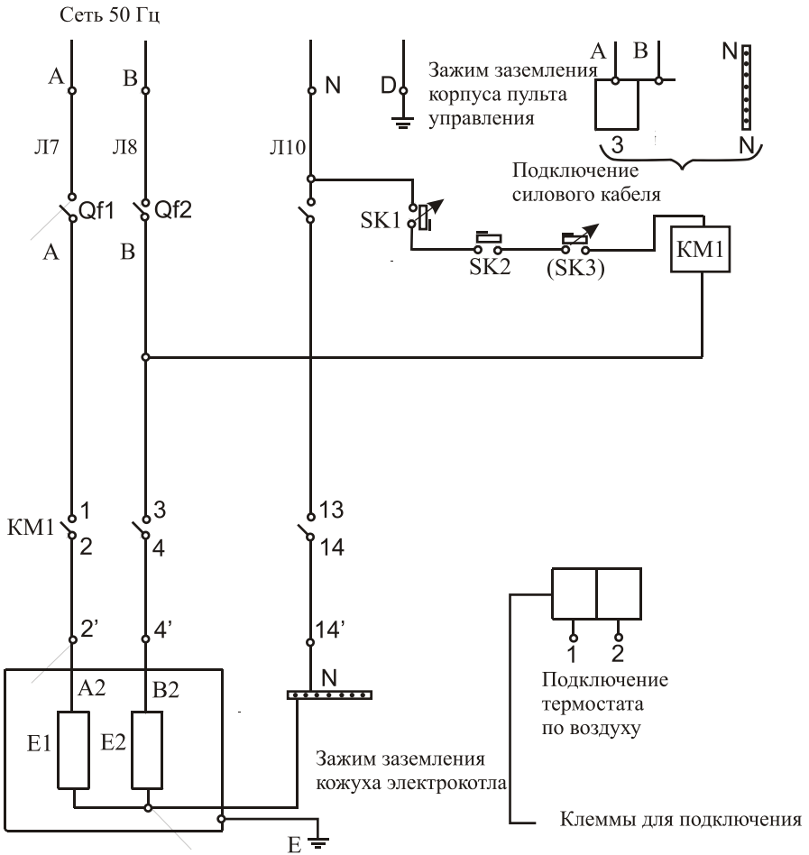
Рис.3 Обозначения к принципиальной электрической схеме пульты управления (продолжение).
